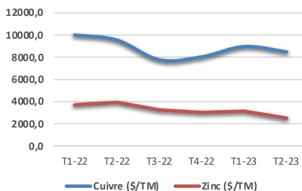
Graphique 3 : Cours du cuivre et du zinc (en dollar/tonne métrique)
