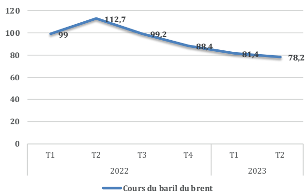
Graphique 1 : Cours du baril du pétrole (en dollar US/baril)
