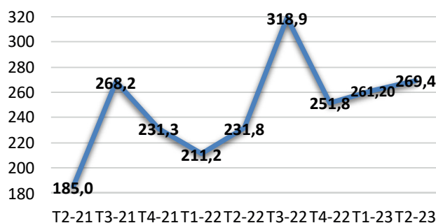
Graphique 11 : Évolution trimestrielle du trafic de passagers (en milliers de personnes)
