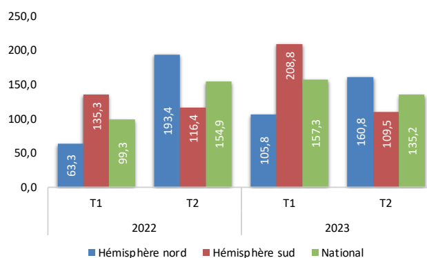
Graphique 14 : Évolution des précipitations (moyenne mensuelle en mm)
